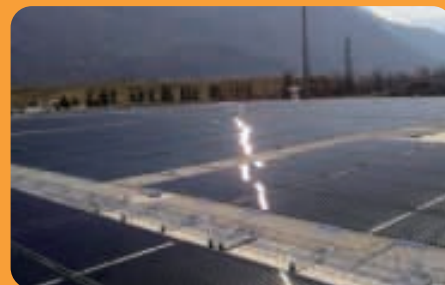
COPERTURA GRANDE DISTRIBUZIONE CON TECNOLOGIA SOLYNDRA 400 kWp
